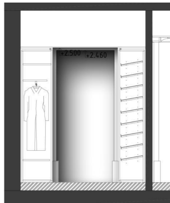
ELEVATION G
