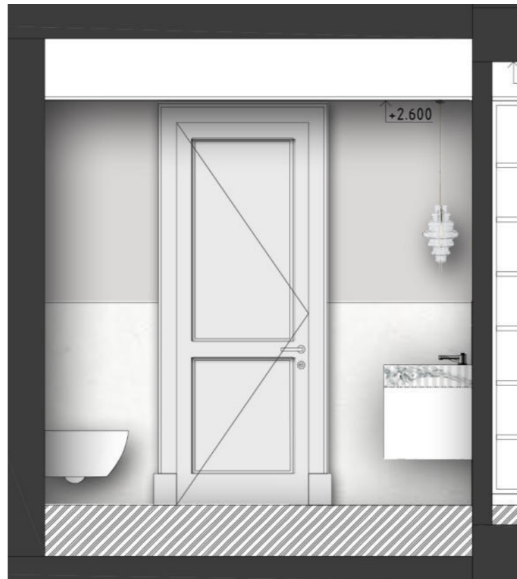
ELEVATION B
